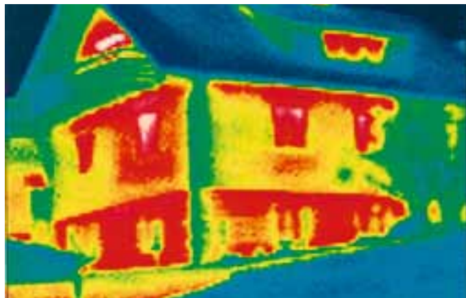
Termografska slika prikazuje konstrukcijske slabosti, kao što su toplotni mostovi, gubitak toplote prema vani.
